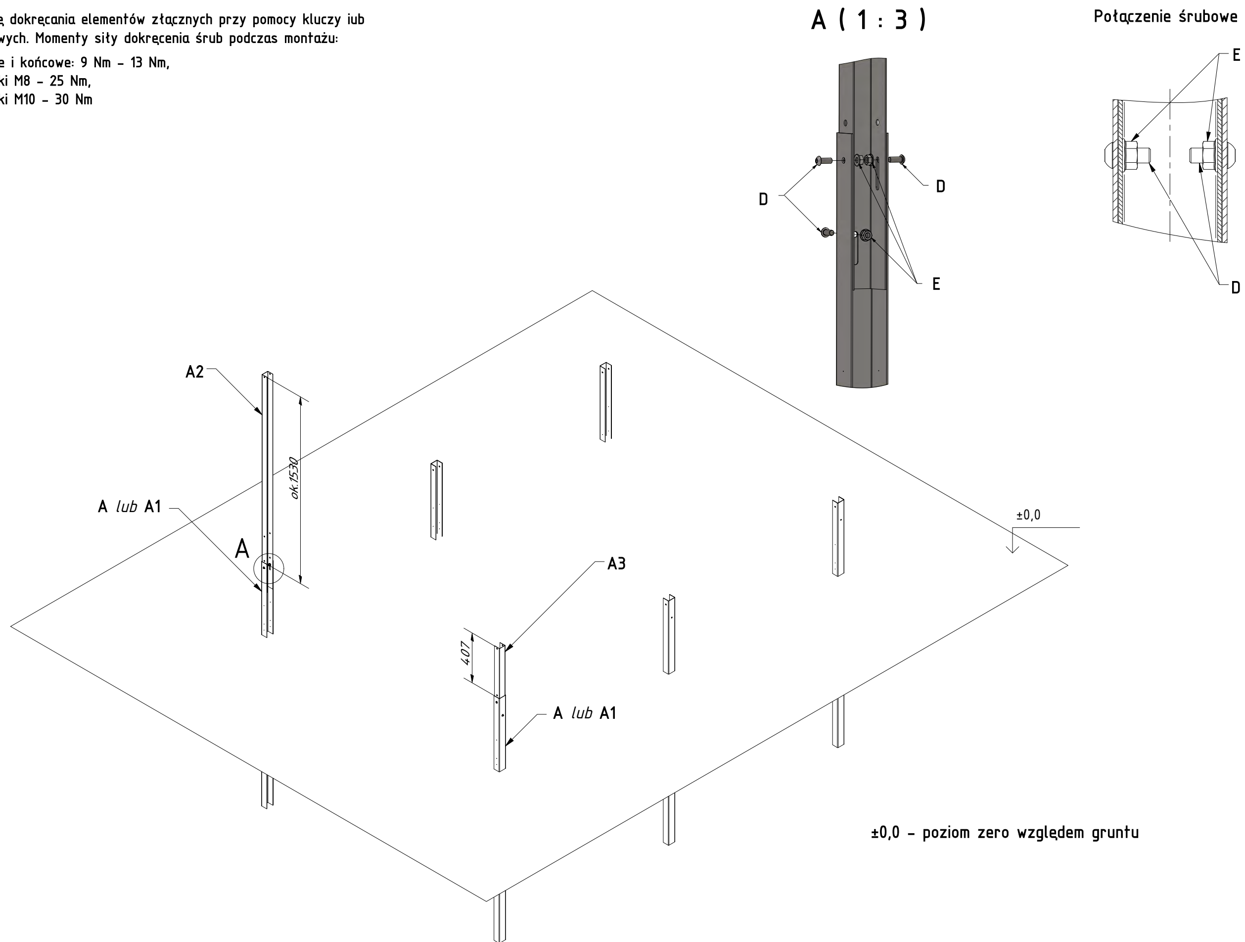
Rys.2-2 Złączenie nóg A (lub A1) z dostawianą nogą tylną (A2) i przednią (A3)
