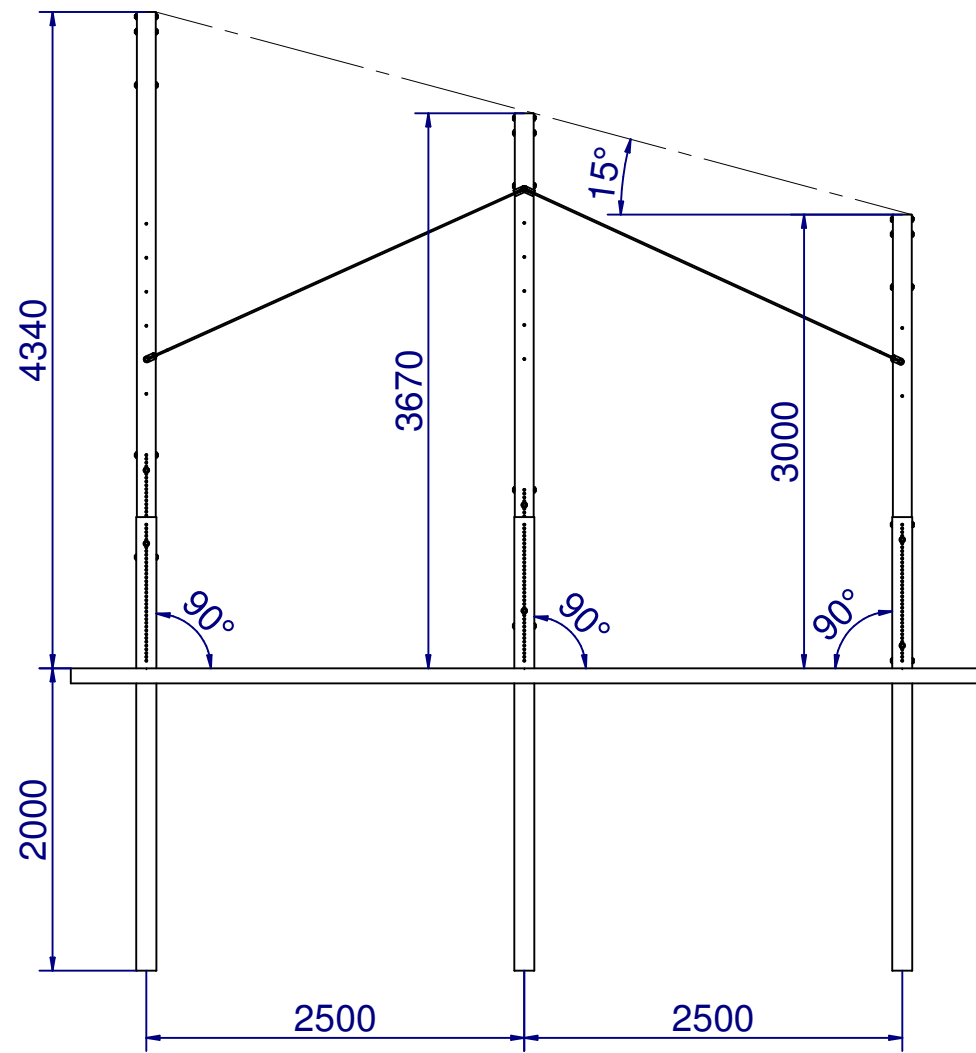
WYMIARY DLA 15°
