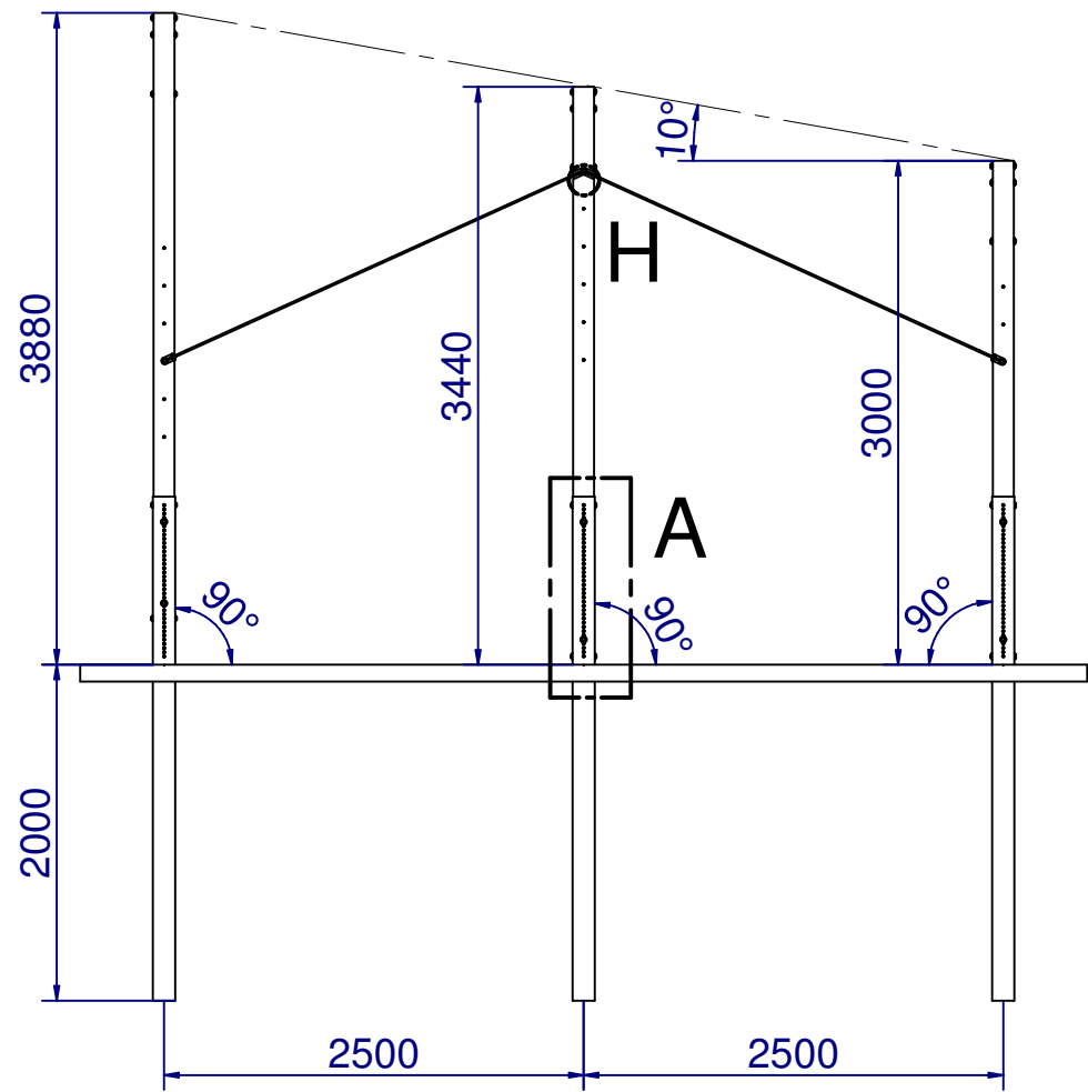
WYMIARY DLA 10°
